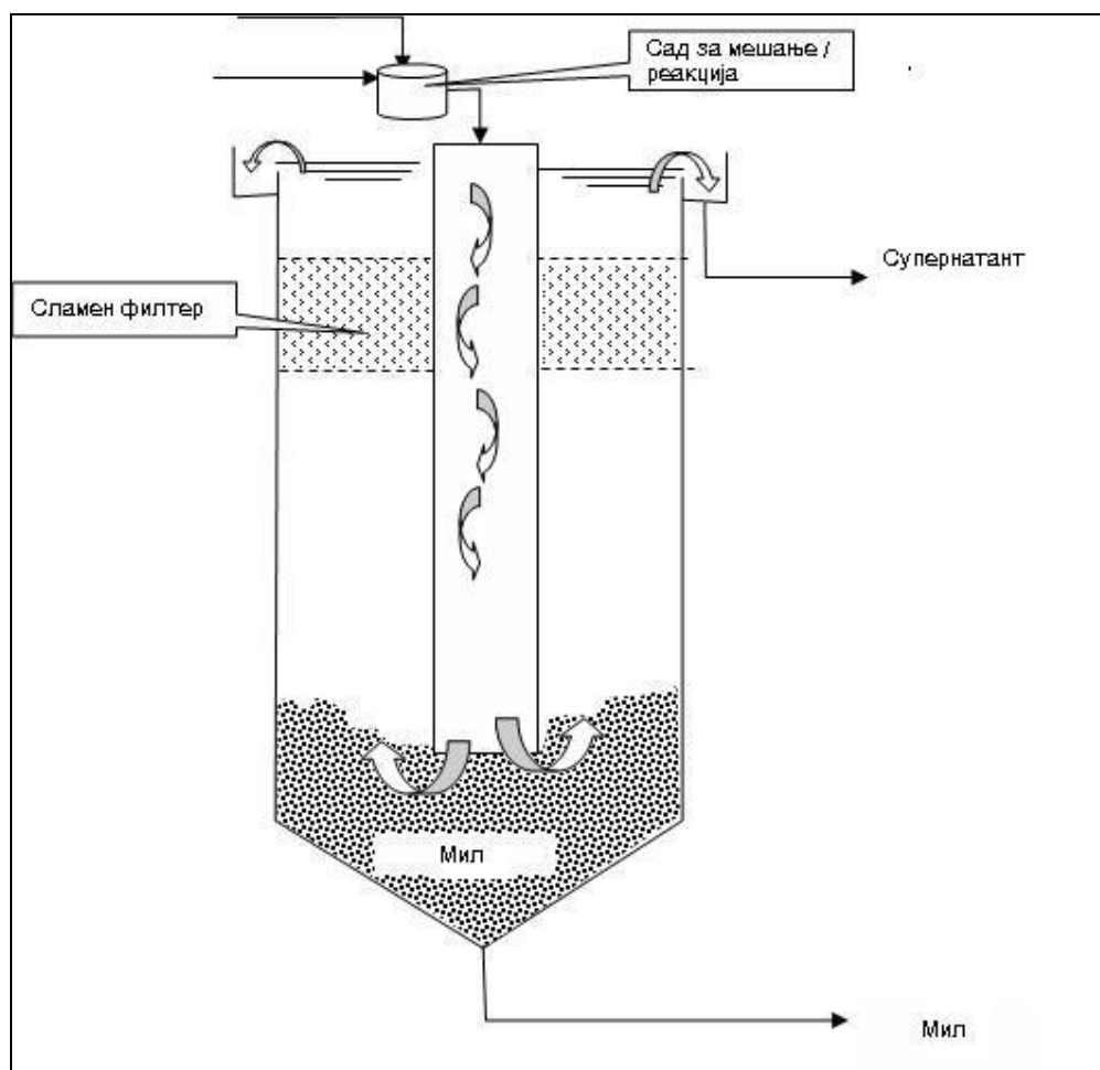
Слика 10 Преципитатор
